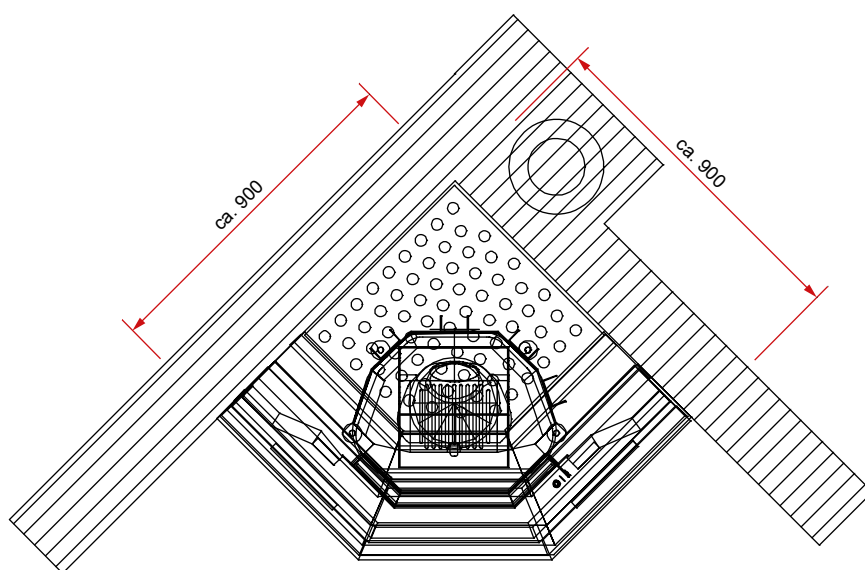
Изображение сверху М 1:20
