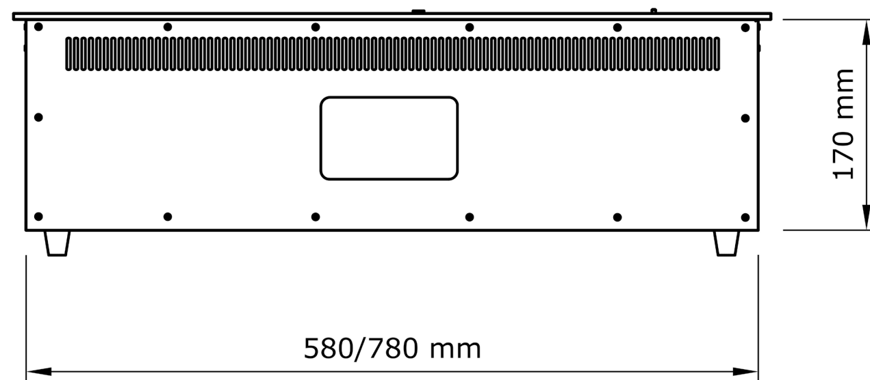
Чертеж корпуса биокамина, габаритные размеры.
