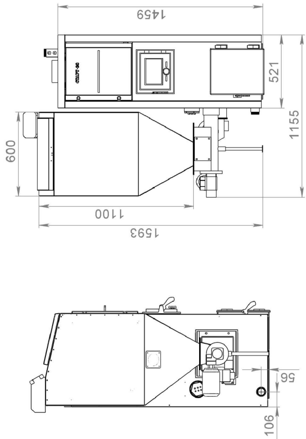
Пеллетный котел "СТАРТ-30-GR-V1", бункер 300 литров
